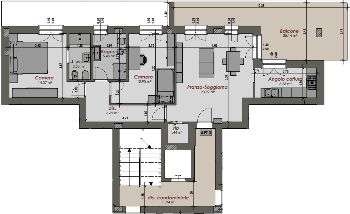
Appartamento 3 Piano Primo Scala 1:100
